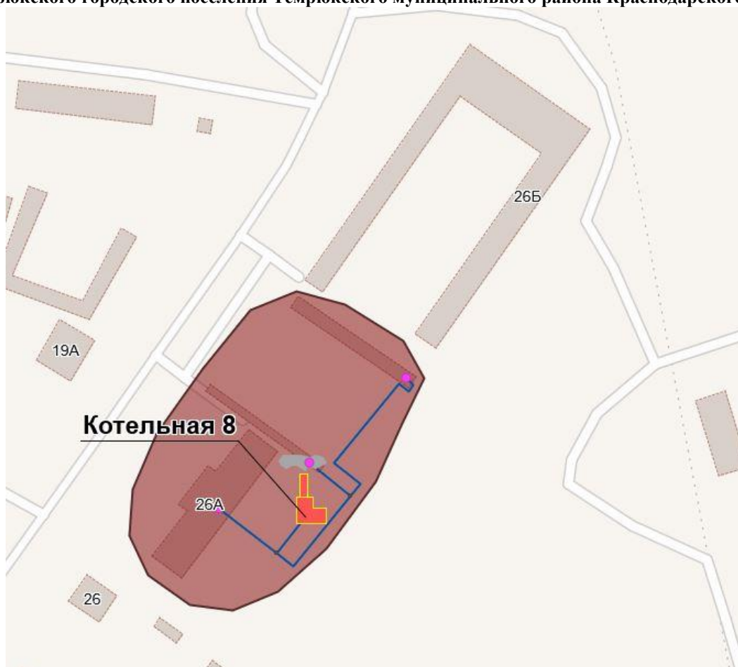
Рисунок 10 Зона действия источника централизованного теплоснабжения (Котельная №8 г. Темрюк, Чуянова, 26к (ТКУ-300) Темрюкского городского поселения Темрюкского муниципального района Краснодарского края
